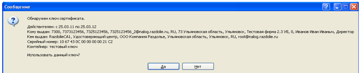
Рис.5. Выбор сертификата
